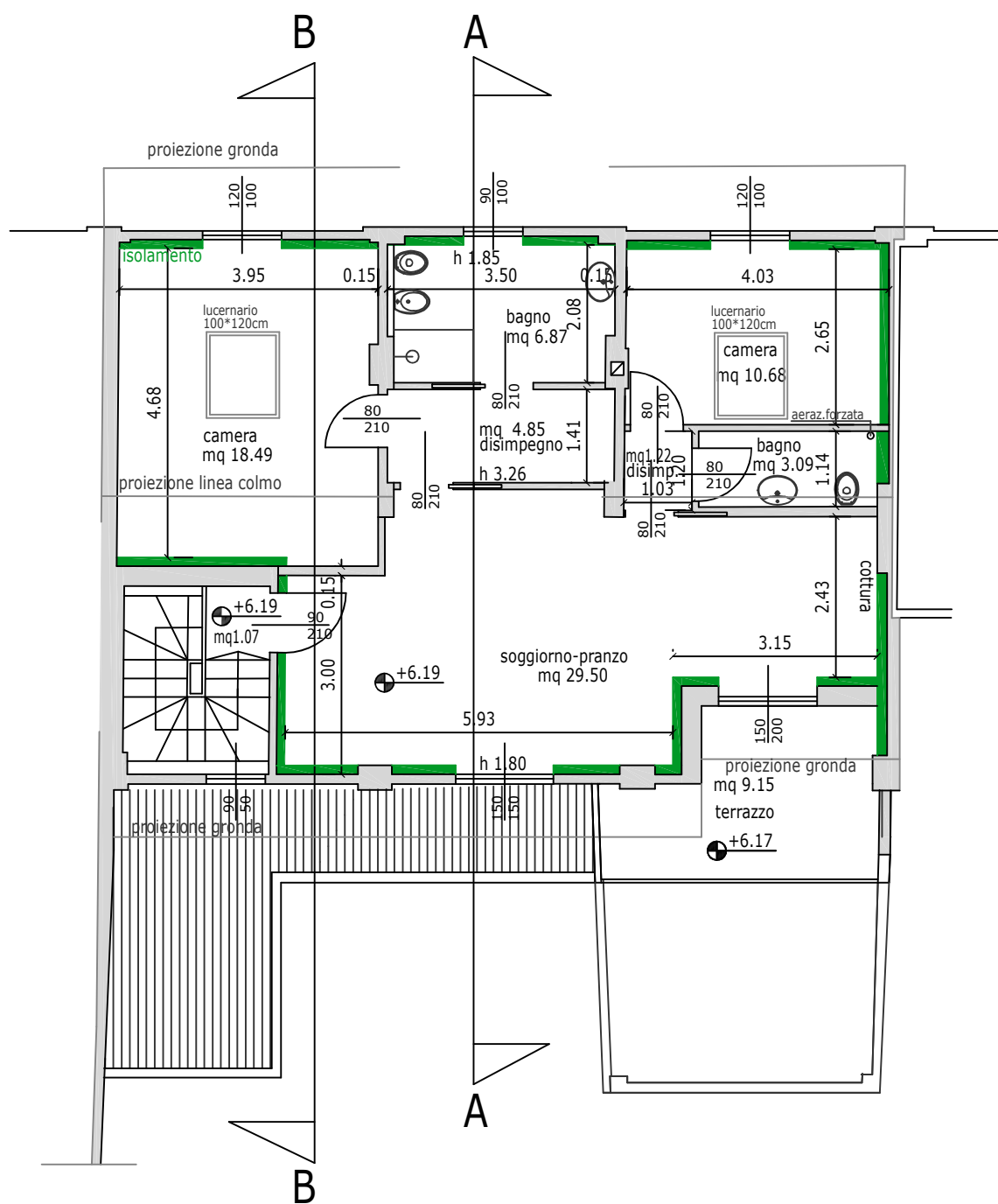
PIANTA PIANO SECONDO - SOTTOTETTO
